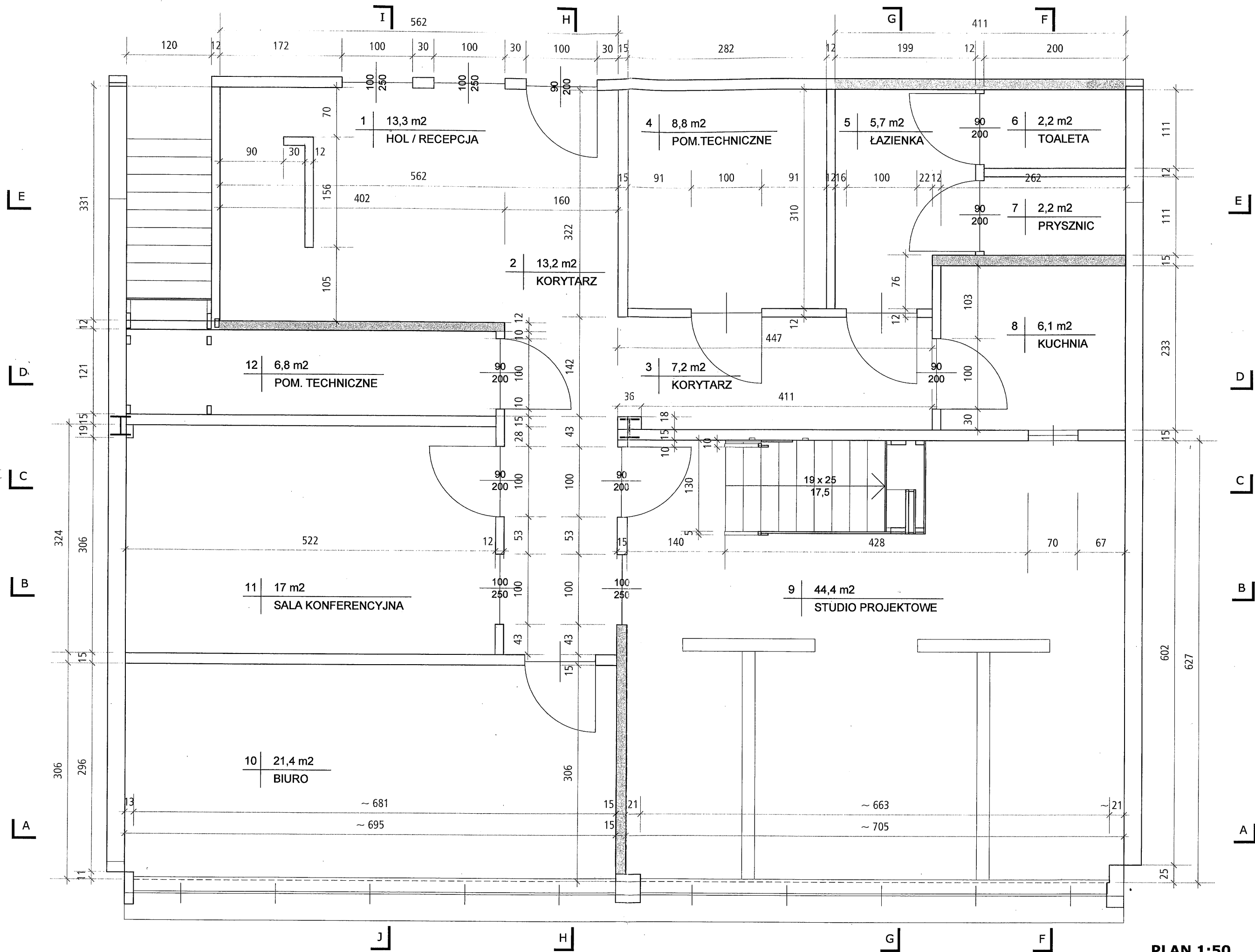
PLAN 1:50
